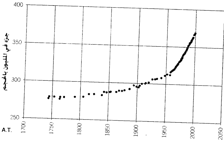
(شكل ١٣-٤) تركيز ثاني أكسيد الكربون في الغلاف الجوى
